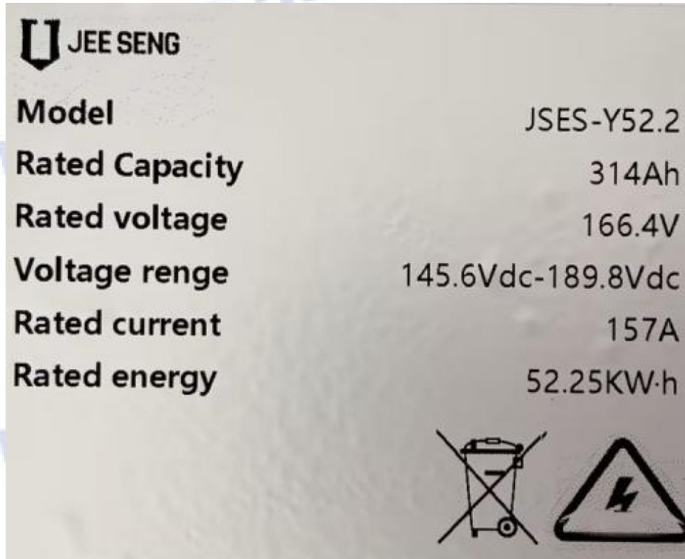
Photo 5 铭牌 Label
